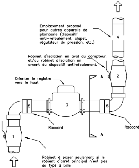
VUE DE FACE (Aucune échelle)
